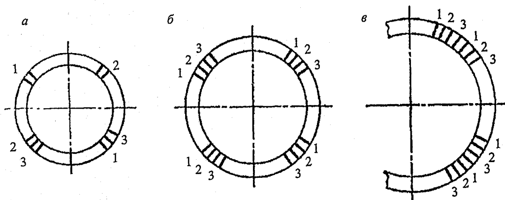
а – трубы диаметром до 400 мм включительно; б – трубы диаметром от 400 до 1000 мм; в – трубы диаметром 1000 мм и более
