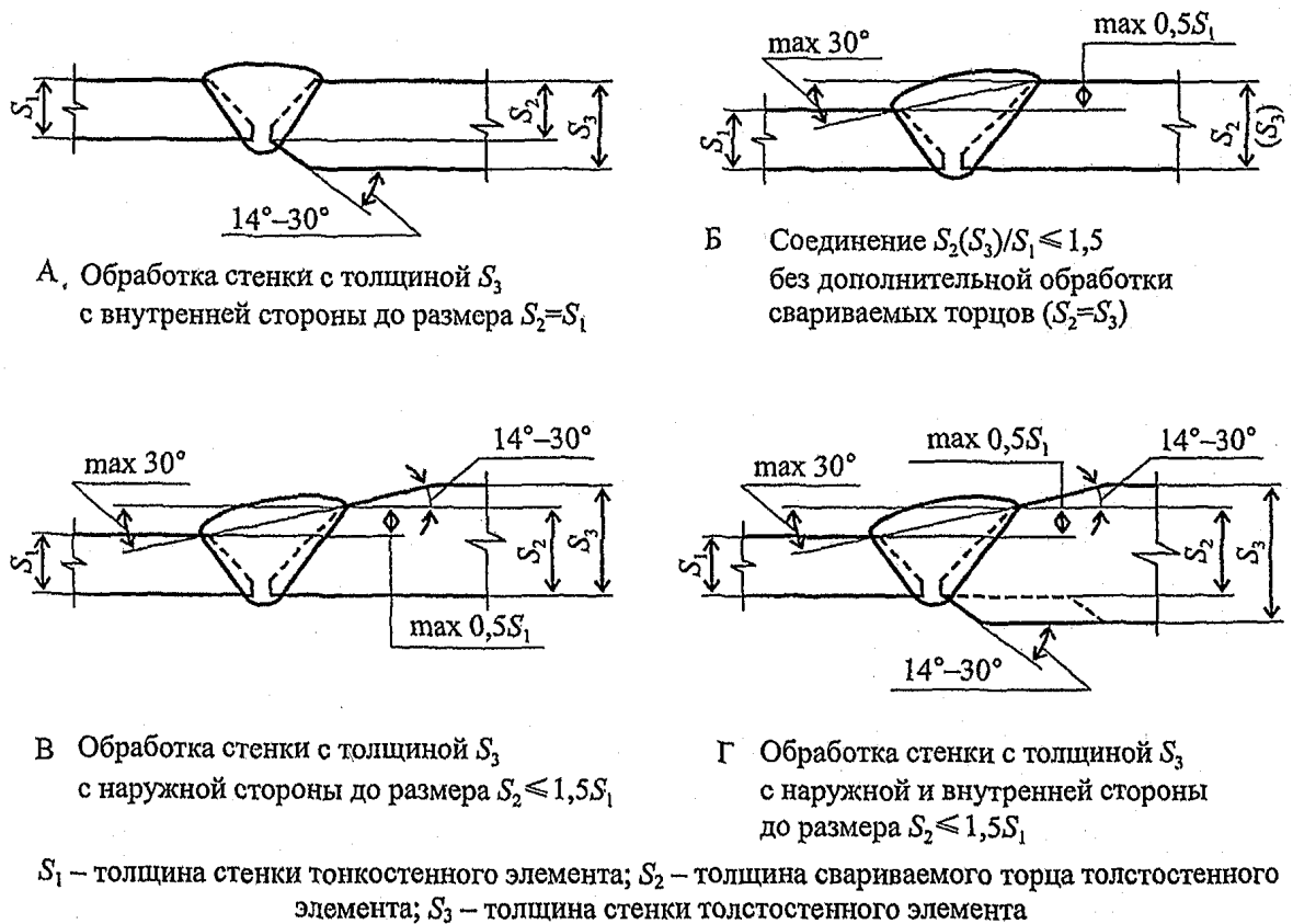
Рисунок 9.2 – Регламентируемые варианты обработки торцов стыкуемых разнотолщинных элементов
